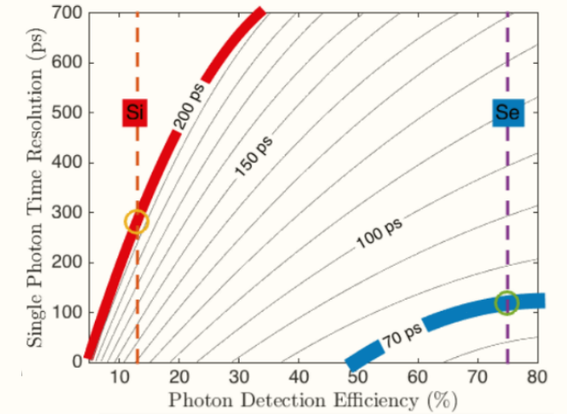
SPTR vs. PDE for Si and a-Se.
